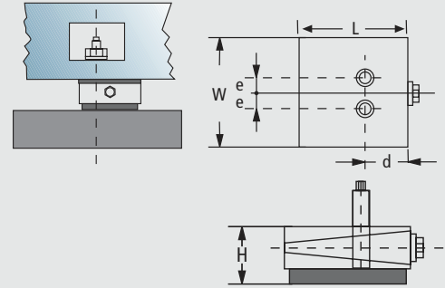
Gildemeister NEF 330 on precision leveling wedges
